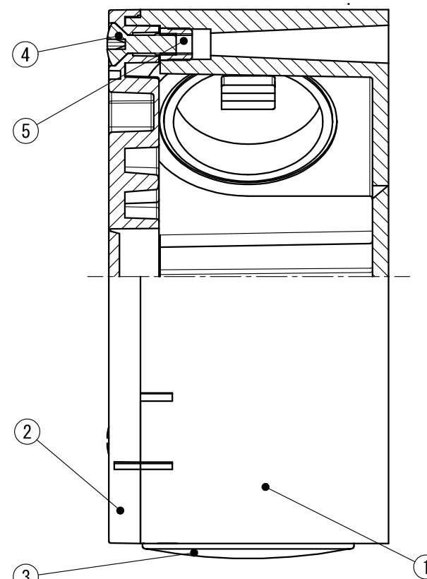
A-A断面図
